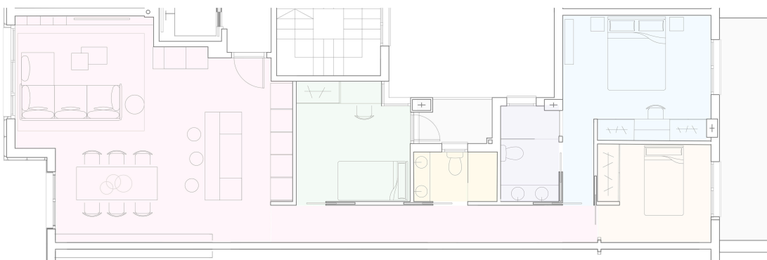
Vivienda TIPO 2 6 viviendas disponibles. Pisos 1-6 * Sin terraza delantera
